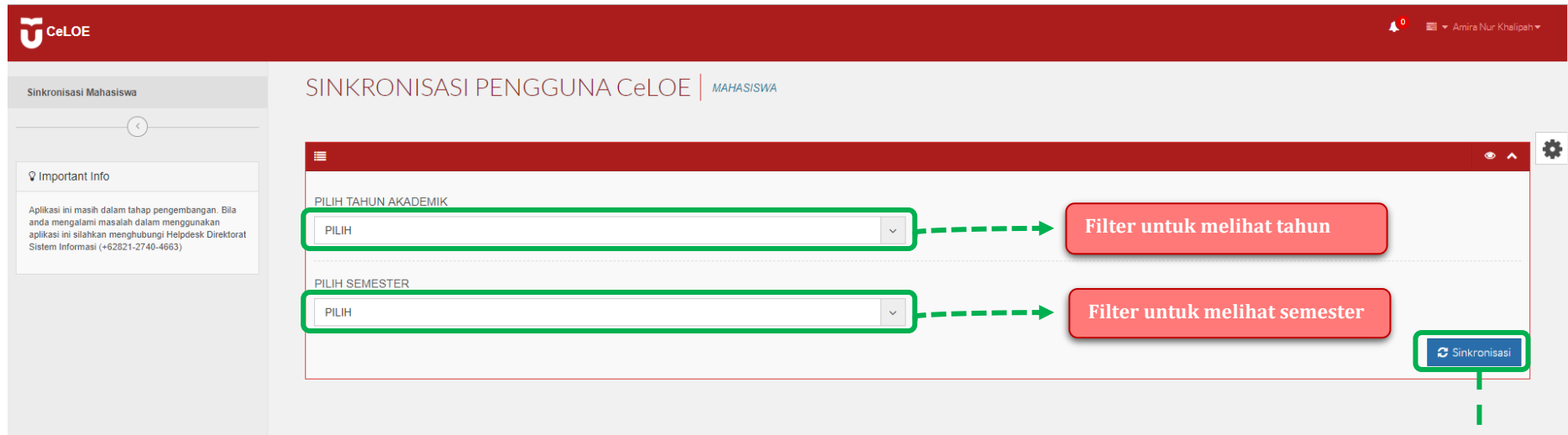
Gambar 3 Administrasi CeLOE
