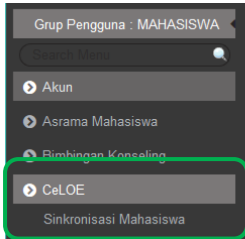
Gambar 2 Menu CeLOE
